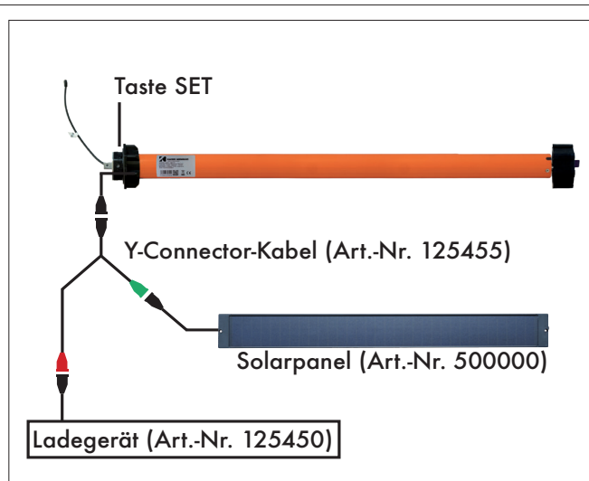
Abb.1: Anschlussbeispiel Favorit Easyline
